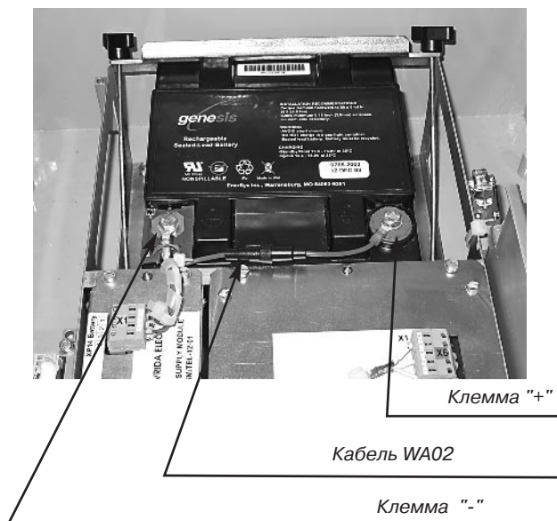
Рис. 4.3. Установка аккумуляторной батареи
