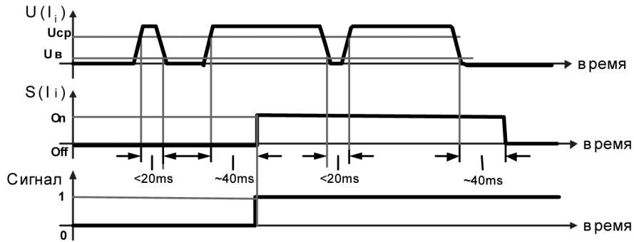
Рис. 3.35. Функционирование входа МДВВ
