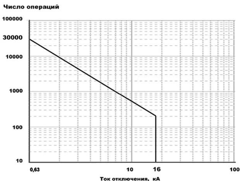
Рис. 2.1. Диаграммы коммутационного ресурса РВА/TEL
