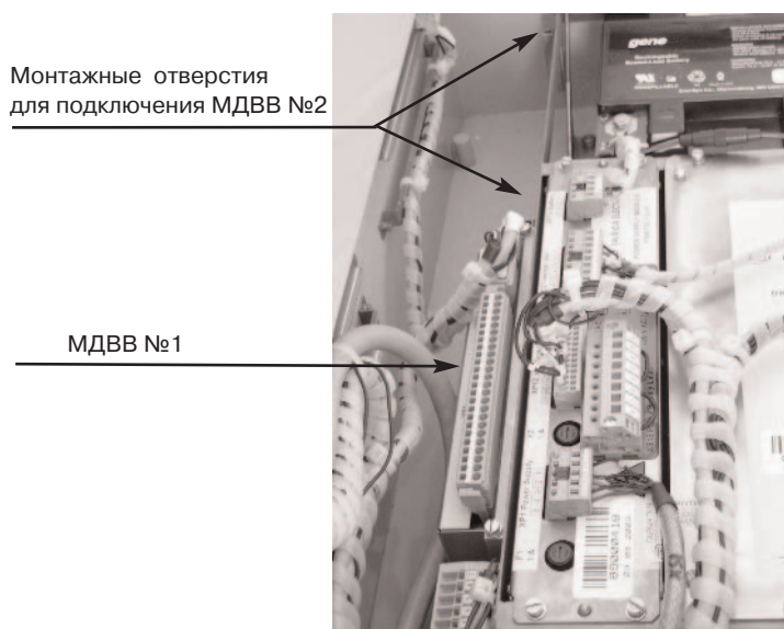
Рис. 3.21. Установка МДВВ в шкафу управления
