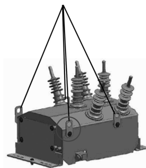
Рис. 4.24. Подъем коммутационного модуля
