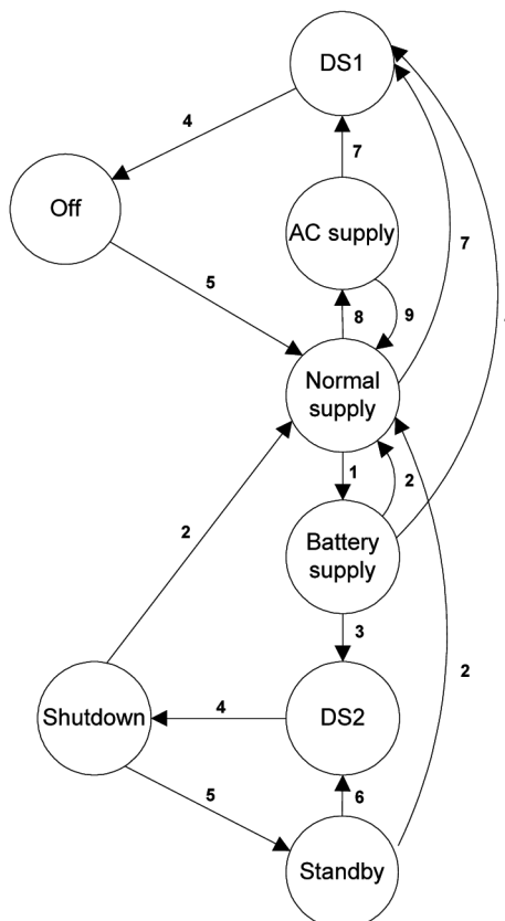
Рис. 3.25. Режимы работы системы бесперебойного питания
