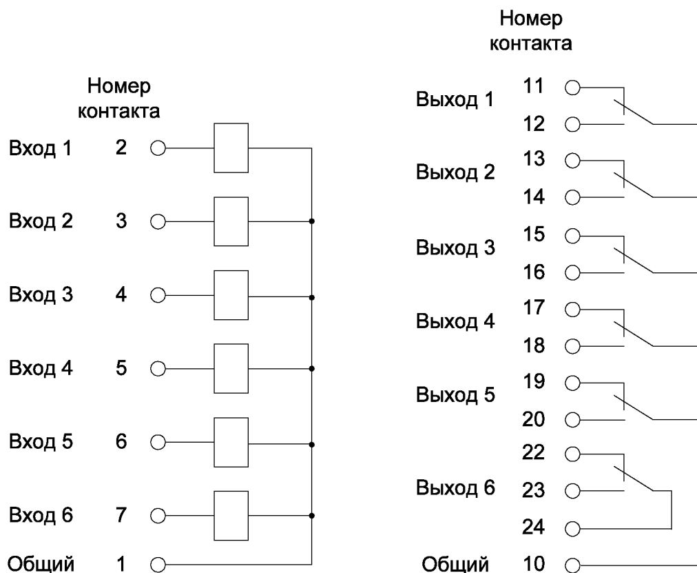
Рис. 3.22. Маркировка дискретных входов и выходов
