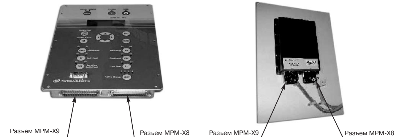
Рис. 3.17. Модуль микропроцессора
