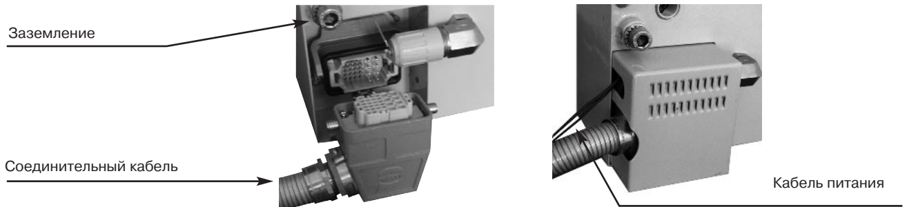
Рис. 3.13. Подключение соединительного кабеля и кабеля питания
