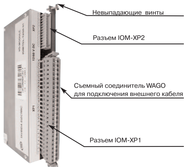
Рис. 3.20. Модуль дискретных входов/выходов
