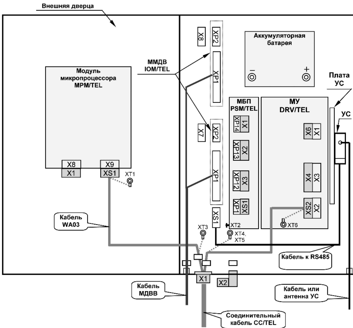
Рис. П3.2. Схемы соединения модулей шкафа управления
