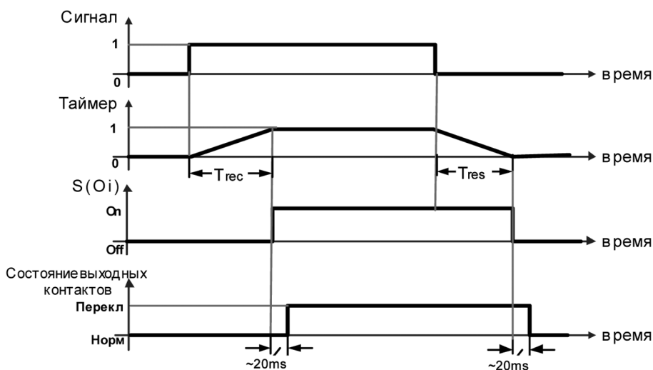
Рис. 3.36. Функционирование выхода МДВВ
