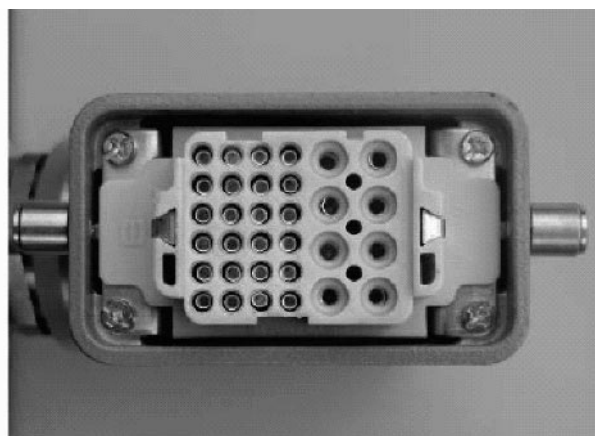
Рис. П4. Разъемы соединительного кабеля СС/TEL со стороны OSM/TEL (слева) и RC/TEL (справа)
