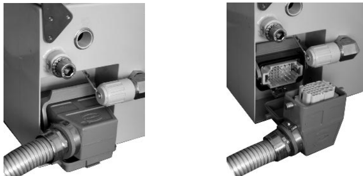
Рис. 4.20. Подключение соединительного кабеля СС/TEL
