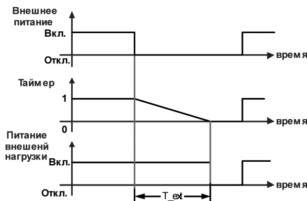
Рис. 3.26. Питание внешней нагрузки
