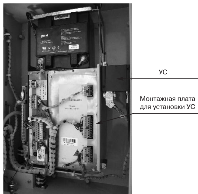
Рис. 3.23. Установка УС
