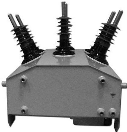
Рис. 3.5. Монтажные отверстия и отверстие под болт заземления
