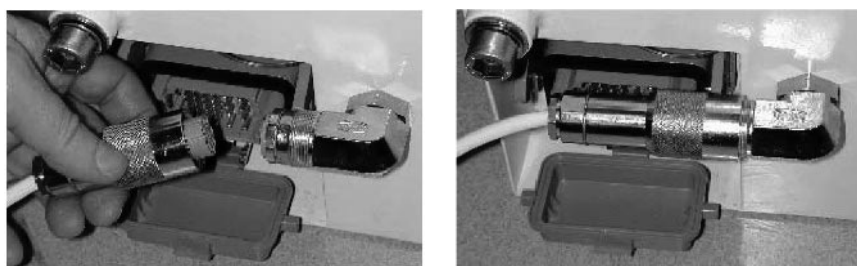
Рис. 4.19. Подключение внешнего оперативного питания
