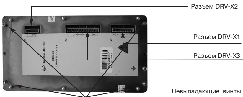
Рис. 3.18. Модуль управления
