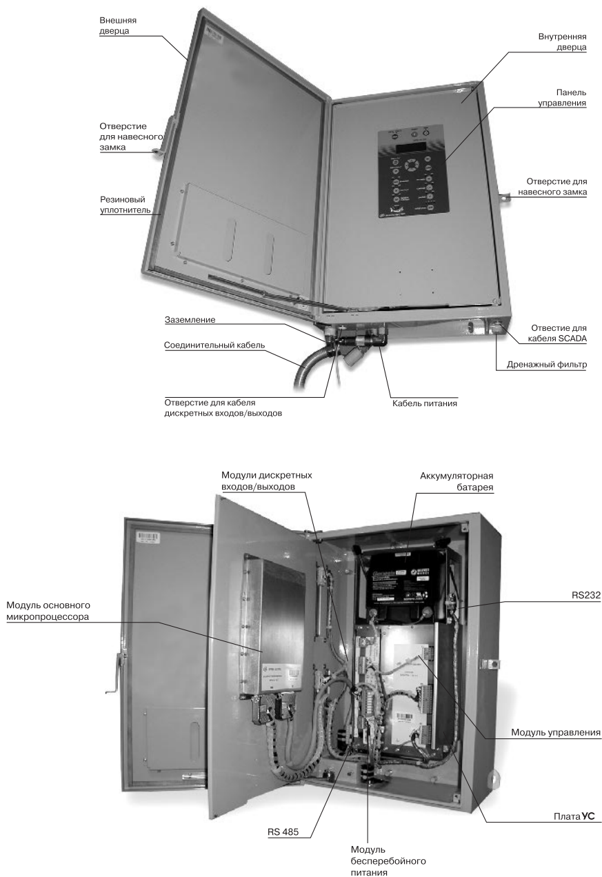
Рис. 3.12. Внешний вид шкафа управления
