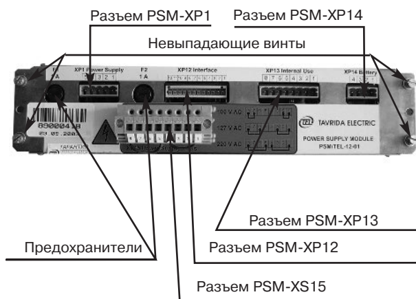
Рис. 3.16. Модуль бесперебойного питания
