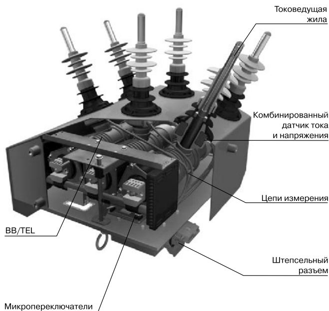
Рис. 3.3. Внутреннее устройство коммутационного модуля
