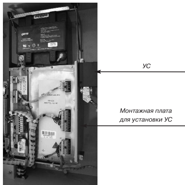
Рис. 4.4. Установка устройства связи со SCADA-системой
