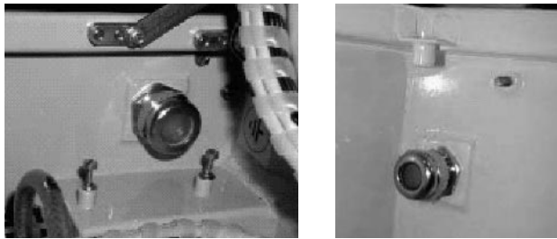
Рис. 3.14. Отверстия для кабелей коммуникаций
