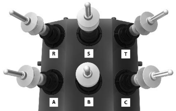
Рис. 3.7. Высоковольтные вводы
