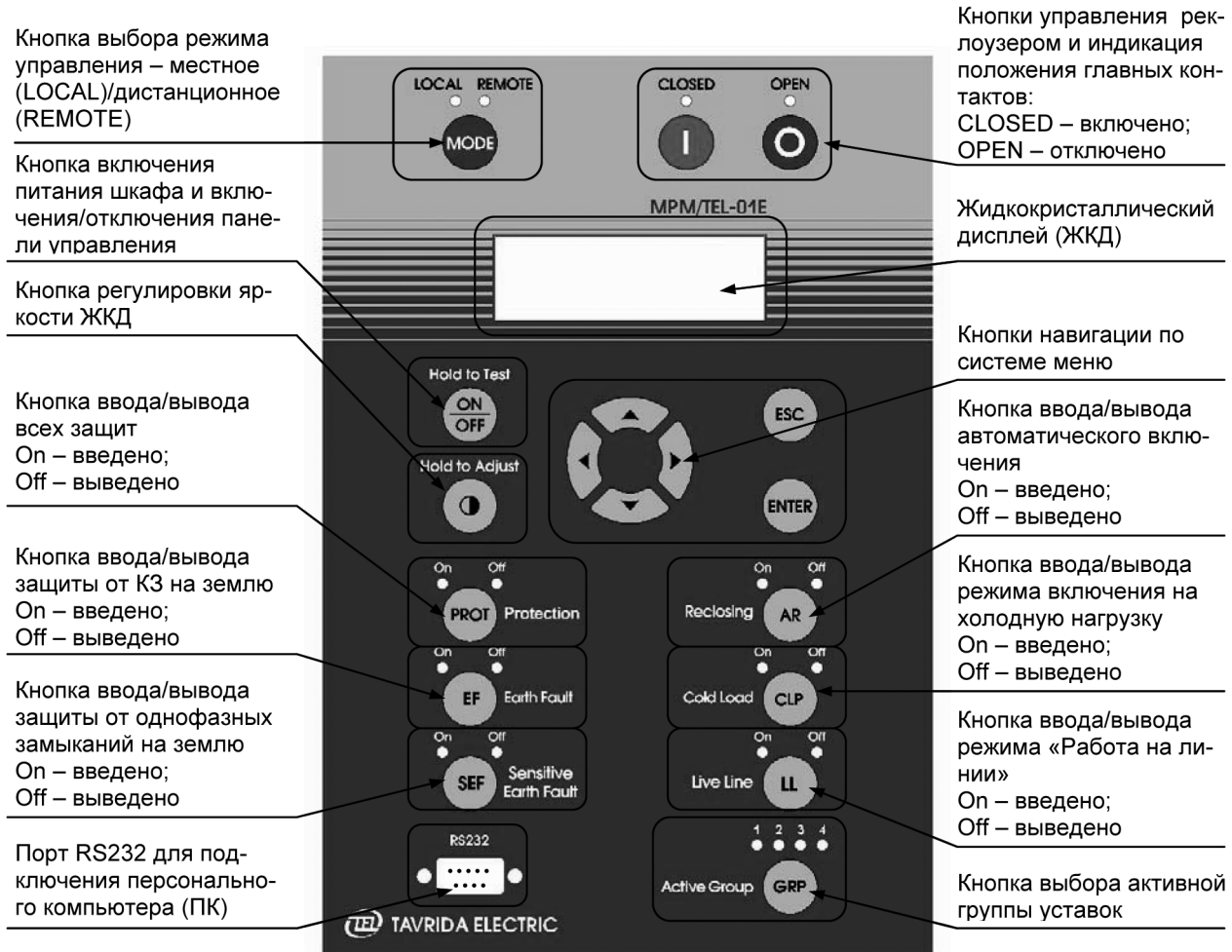
Рис. 3.28. Панель управления шкафа управления
