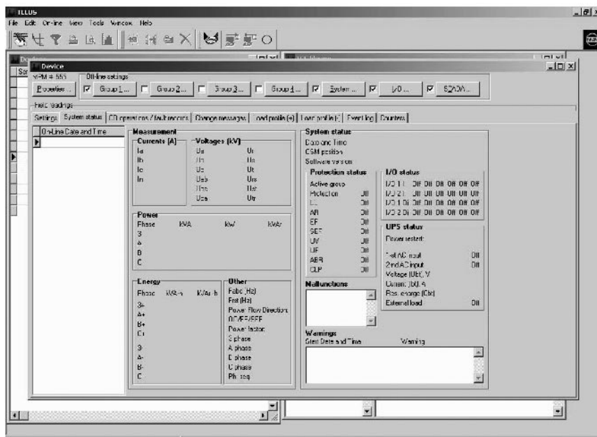
Рис. 4.21. Окно Devices реклоузера
